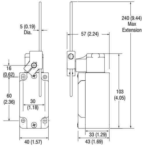
Rod Lever
