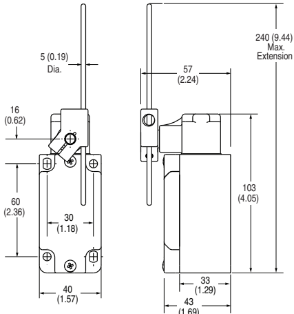
Rod Lever
