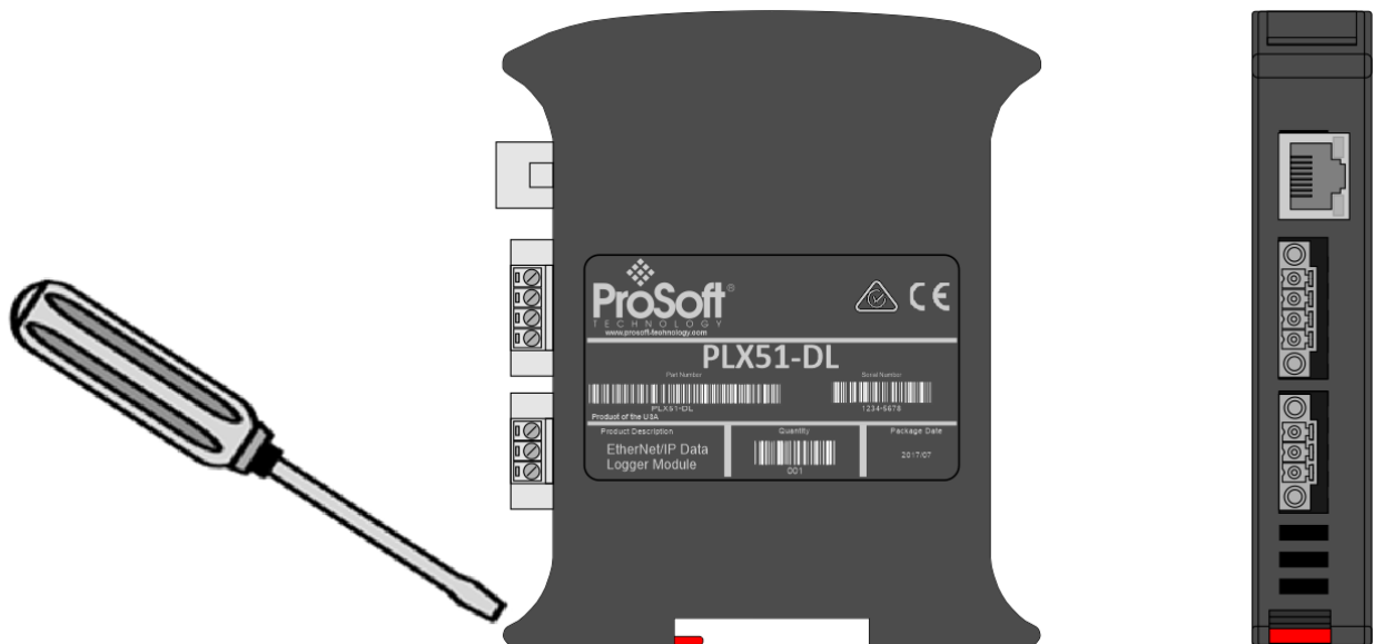
Figure 2.4. - DIN rail mounting
